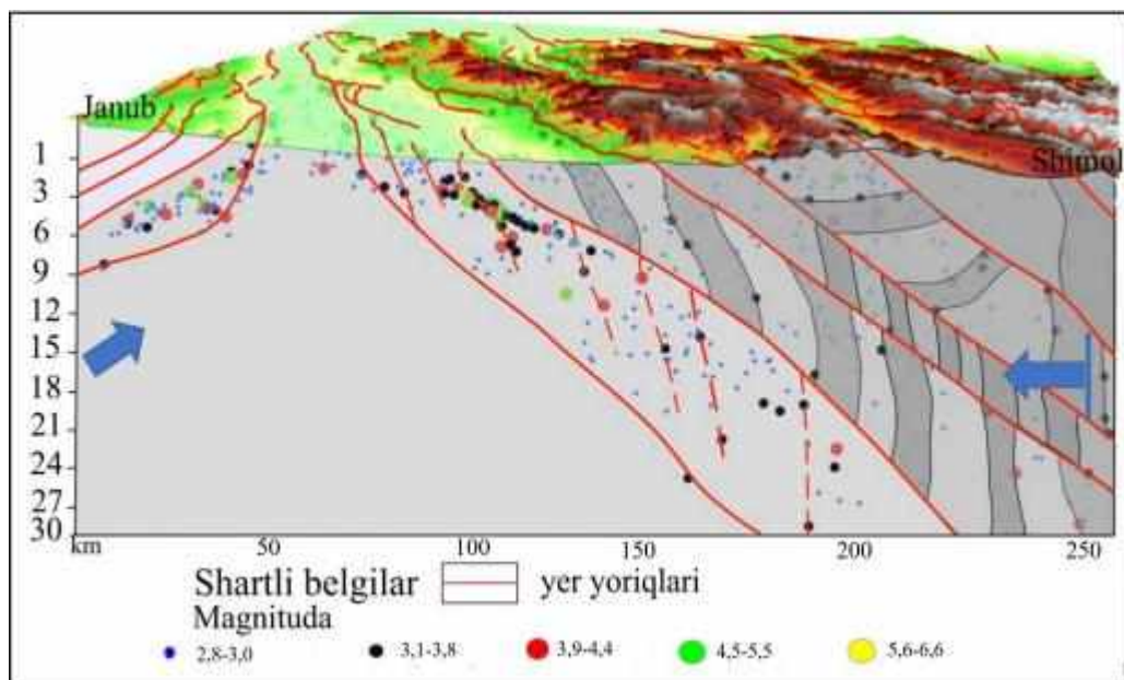
4-rasm. Chotqol-Qurama (Tovoqsoy poligoni) hududining zilzilalar katalogi asosida yaratilgan yer qobig‘ining geodinamik modeli
