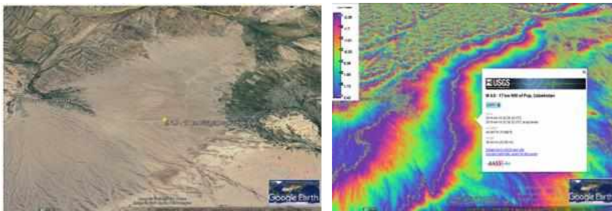
3-rasm. Radarli interferometriya usuli orqali zilzila kuchi qiyosiy baholash natijasi va yer qobig'ining zamonaviy vertikal harakatlari
