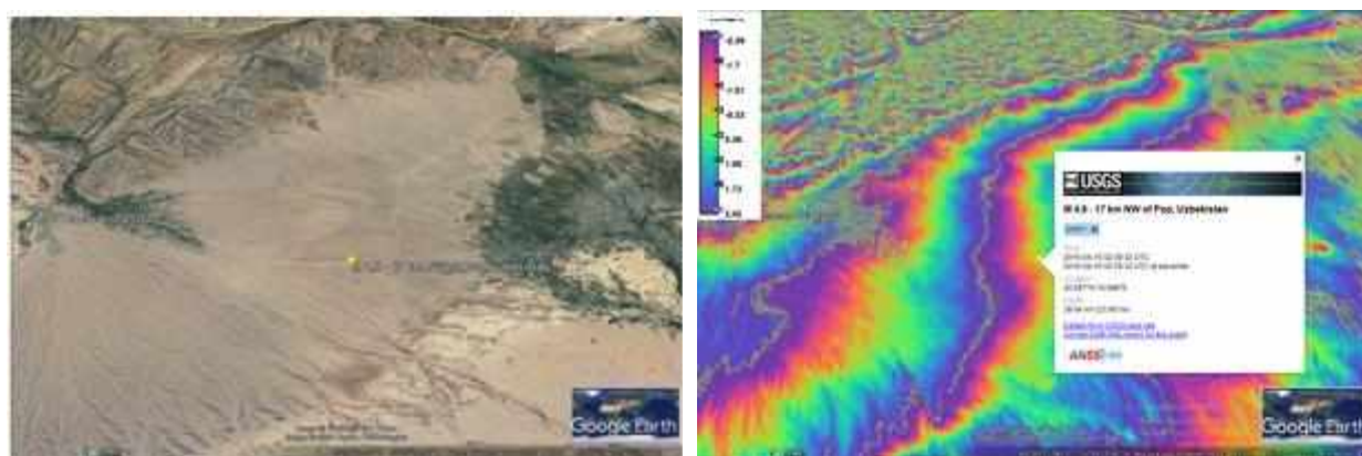
Рис.3. Результат сравнительной оценки магнитуды землетрясения и современные вертикальные движения земной коры, определенные методом радарной интерферометрии
