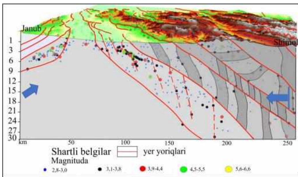
Рис. 4. Глубинная модель земной коры, созданная на основе каталога землетрясений Чаткало-Кураминского района (Таваксайский полигон)
