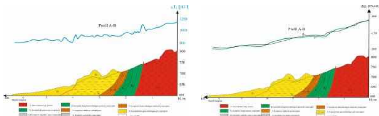
Рис. 1. График геологического разреза и магнитного поля \Delta T а так же график силы тяжести \Delta g_a площади Таваксай по профилю АВ
