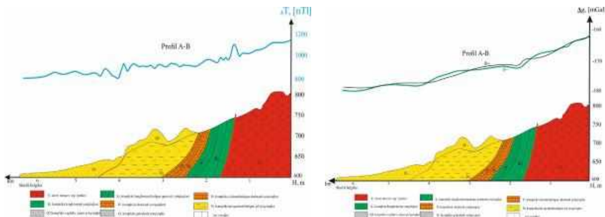
1-rasm. Tovoqsoy maydonining AB profil bo'yicha geologik kesim va magnit maydon \Delta T grafigi hamda og'irlik kuchi \Delta g_a grafigi
