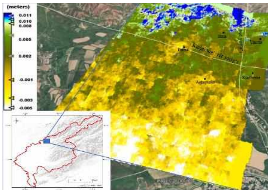
2-rasm. Radarli interferometriya usulida qayta ishlash natijasida aniqlangan yer qobig‘ining vertikal harakatlari (mm)
